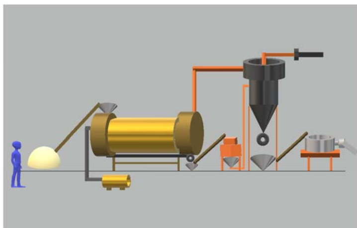
Рис.1. 3Д-модель схемы размещения линии производства гранул
